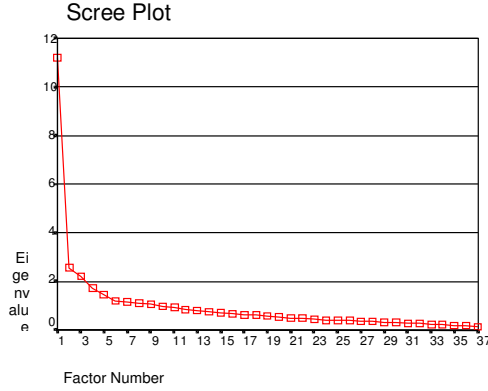
شكل رقم (1) التمثيل البياني للعوامل (Scree Plot)
