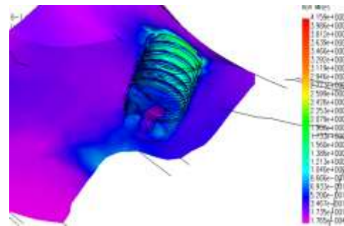
الشكل (4) : تركيز الإجهادات عند العنق، وتناقصها التدريجي على طول الزرعة
