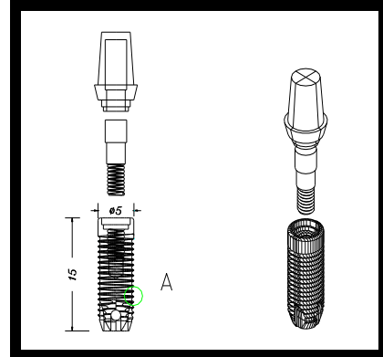
الشكل (2) : نموذج الزرعة السنية والدعامة ويرغي التثبيت
